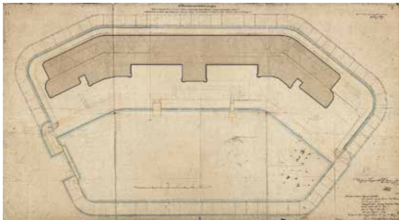
Ил. 19. План острова Константиновской батареи «... с изображением на оном пунктирными линиями очерка предполагаемой в последствии времени каменной батареи». Январь 1859 г. Упомянутые пунктирные линии на оригинальном чертеже едва различимы. Поэтому здесь они дополнительно обведены, а площадь каменного здания батареи залита темным тоном. РГАВМФ. Ф. 1341. Оп. 4. Д. 3886
