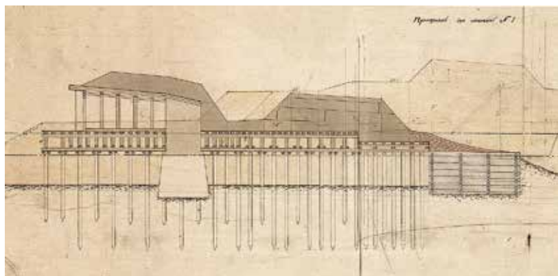
Ил. 23. Фрагмент разреза к проекту перестройки временной батареи № 1. На чертеже темной заливкой показаны временные сооружения, построенные в первой половине 1863 года. Слева блиндированное помещение, напольная стена которого, имеет фундамент, опирающийся на дно залива. Справа — ряжевая эскарпная стенка. РГАВМФ. Ф. 1341. Оп. 4. Д. 4595
