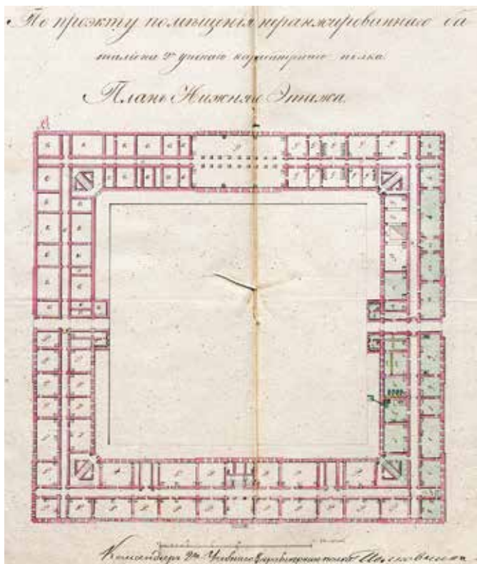
Ил. 4. Проект помещений неранжированного батальона 2-го Учебного карабинерного полка. План нижнего этажа. РГВИА. Ф. 405. Оп. 5. Д. 7546. Л. 35-46 об.
