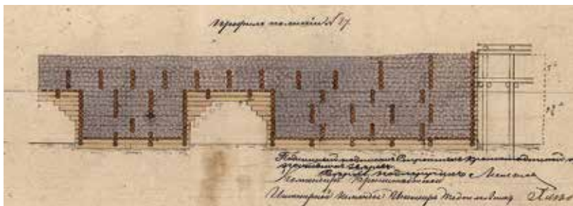
Ил. 20б. «Чертеж морской батареи № 6 ...» Фрагмент с разрезом по ряжевому молу, построенному в 1859 и 1860 годах
