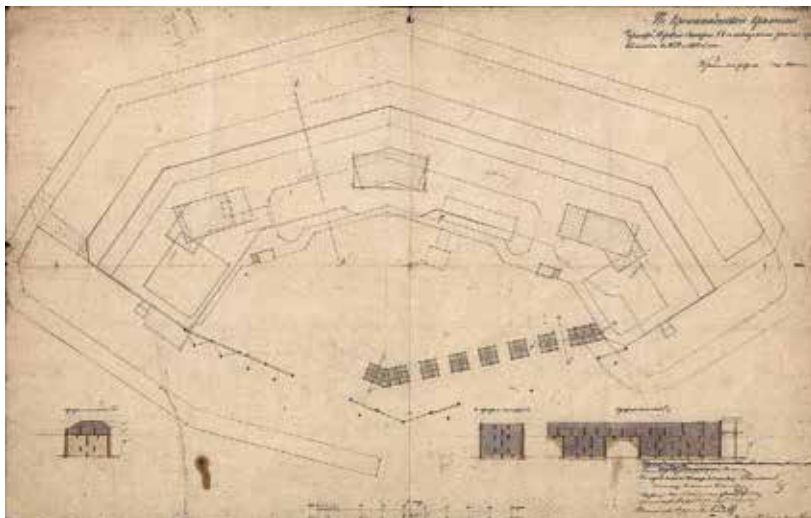
Ил. 20а. «Чертеж морской батареи № 6 с показанием работ, произведенных в 1859 и 1860 годах». РГАВМФ. Ф. 1341. Оп. 4. Д. 4309
