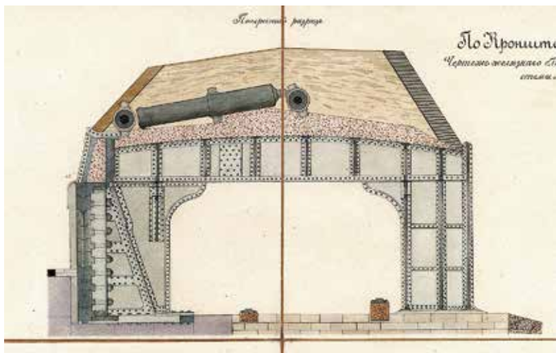
Ил. 28. Броневой брестер Ланкастера, перекрытый в 1870 году железным блиндажом. РГАВМФ. Ф. 1341. Оп. 2. Д. 303
