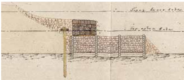
Ил. 22а. Разрез по острову и одноэтажному казематированному traversу морской батареи № 6. К проекту 1861 года. В таком виде проект реализован не был. РГАВМФ. Ф. 1341. Оп. 4. Д. 4312
