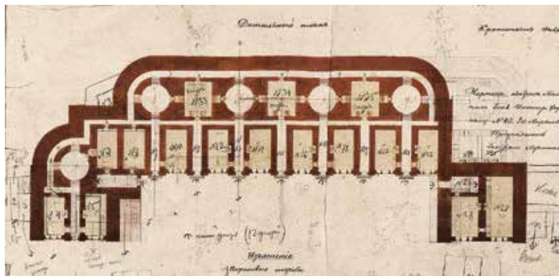
Ил. 39б. План помещений массива башенной батареи к проекту, составленному 27 февраля 1867 г. РГАВМФ. Ф. 1341. Оп. 4. Д. 4852
