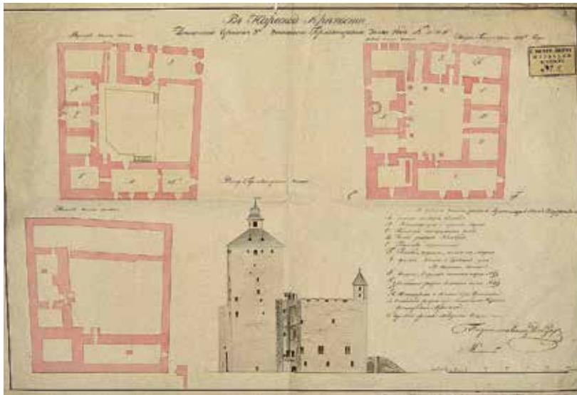
Ил. 2 Ф. 27 К-ка Крепости и Укрепления № 1 Д. 331. Детальный чертеж трехэтажного Гермейстерского замка в Нарвской крепости
