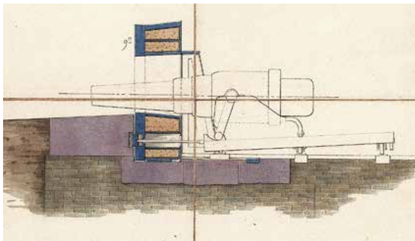
Ил. 44. Разрез по Колпинскому броневому брустверу на пять 11-дм. пушек. РГАВМФ. Ф. 1341. Оп. 2. Д. 305
