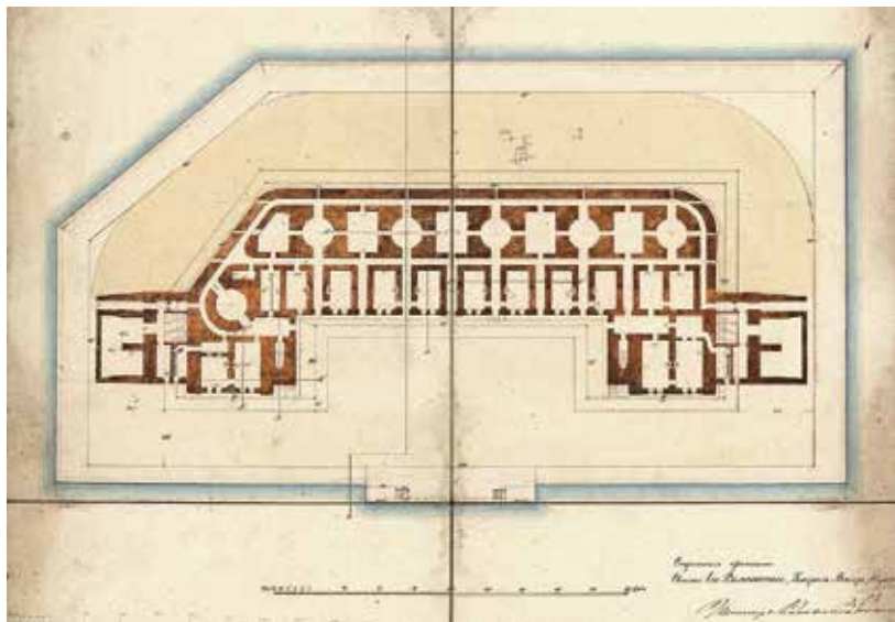
Ил. 51. Окончательный план помещений массива башенной батареи с двумя фланговыми пристройками. РГАВМФ. Ф. 1341. Оп. 4. Д. 6073
