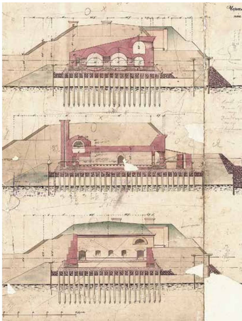
Ил. 46. Разрезы и фасад кирпичного порохового погреба на соединительном участке Константиновской батареи. РГАВМФ. Ф. 1341. Оп. 4. Д. 5302
