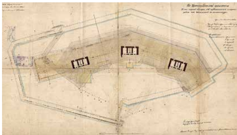
Ил. 21. Проект перестройки временной морской батареи № 6. 28 июля 1861 г. РГАВМФ. Ф. 1341. Оп. 4. Д. 4310
