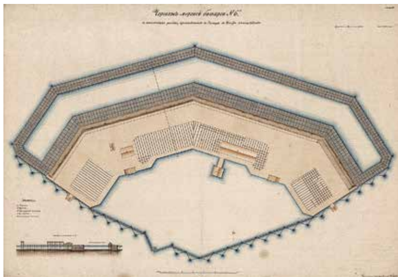
Ил. 13а. План временной морской батареи № 6 выше ординара. 1856 г. РГАВМФ. Ф. 1341. Оп. 4. Д. 3727
