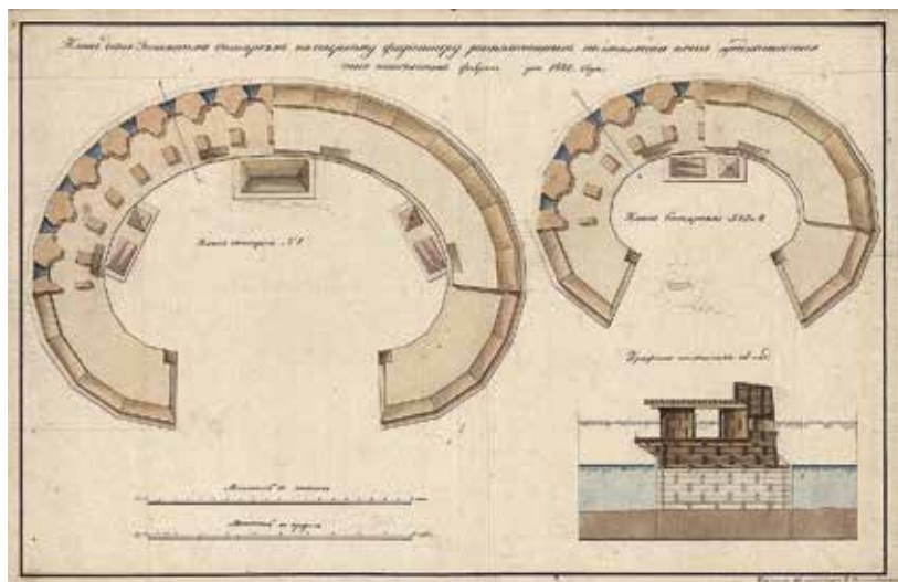
Ил. 5а. «План двух-этажным батареям по северному фарватеру расположенных, по ветхости коих предполагается оные возобновить» 1826 г. РГАВМФ. Ф. 1341. Оп. 4. Д. 1484
