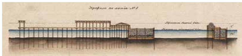
Ил. 13б. Разрез по временной батарее № 6 (фрагмент предыдущего чертежа). В левой части разреза — место без настила, оставленное под блиндированную постройку. Справа — ряжевый волнолом. Чертеж показывает состояние укрепления, после окончания работ в 1856 году
