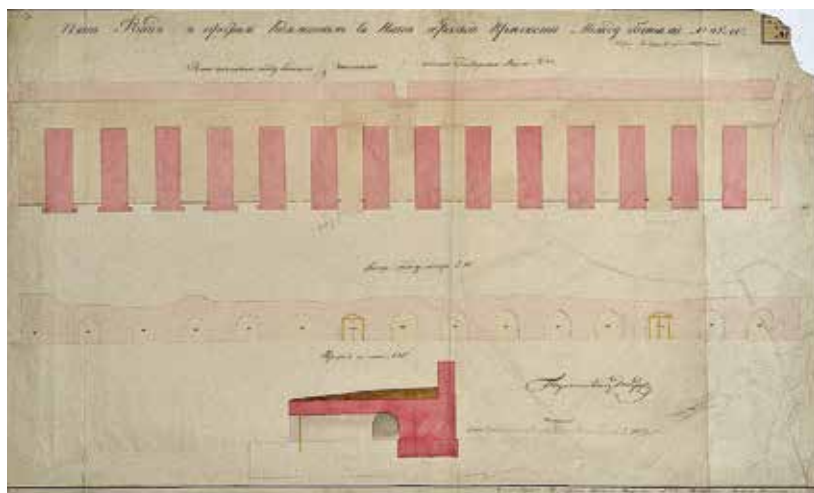
Ил. 1 Ф. 27 К-ка Крепости и Укрепления № 1 Д. 328. План, фасад и профиль казематам в Иван Градской крепости между башнями № 4 и 5
