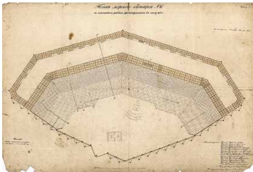
Ил. 12. План временной морской батареи № 6 ниже ординара (по сваям и ряжевым ящикам). 1856 г. РГАВМФ. Ф. 1341. Оп. 4. Д. 3728
