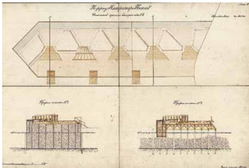
Ил. 17. «По форту Император Павел I. Детальный чертеж батареи под № 3». 1856 г. Кривая линия в правой части плана батареи — абрис горжевой стены форта «Павел I». Левый разрез по ряжевому основанию деревянного капонира, правый по участку между ряжевым основанием и стеной форта (эта часть батареи спроектирована на свайном основании). РГАВМФ. Ф. 1341. Оп. 4. Д. 3824
