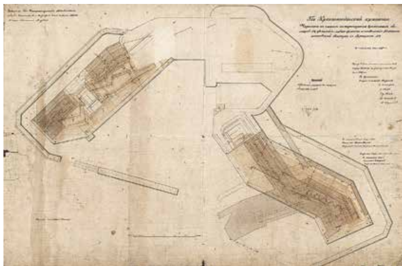
Ил. 47а. «Чертеж к смете по перестройке временных батарей № 4, удлинения левого фланга и соединения Константиновской батареи с батареею № 4». 24 мая 1867 г. РГАВМФ. Ф. 1341. Оп. 4. Д. 4933
