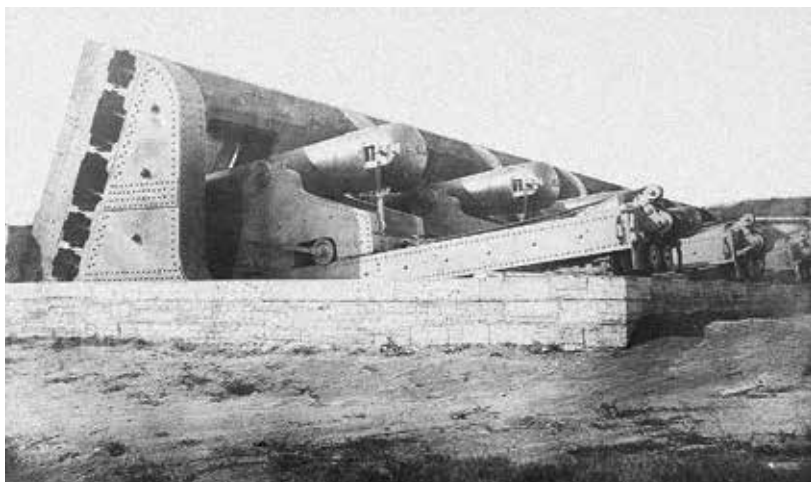
Ил. 27. 8-дм. пушки обр. 1867 г. за 9-орудийным броневым брестером по системе комитета на батарее «Константин». Фото 1869 г. Из фондов ВИМАИВиВС
