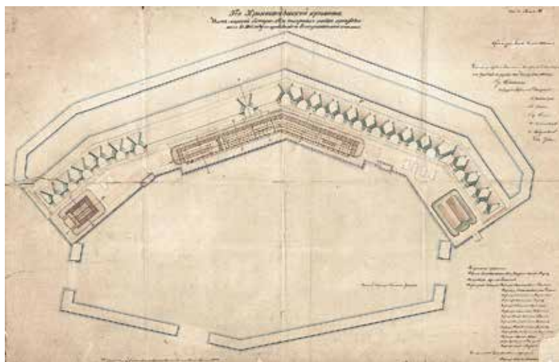
Ил. 24 «План морской батареи № 8 с показанием работ, произведенных в 1863 году по приведению ее в оборонительное положение». Ряжевый мол, огораживающий гавань, был построен в 1859 и 1860 годах. РГАВМФ. Ф. 1341. Оп. 4. Д. 4880
