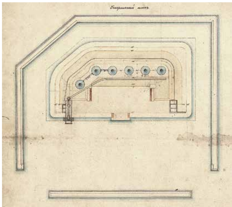
Ил. 50а. Проект морской батареи на 17 орудий в шести броне-вых башнях и за двумя участками броне-вых брустверов. 12 апреля 1869 г. Генеральный план. РГАВМФ. Ф. 1341. Оп. 4. Д. 6074
