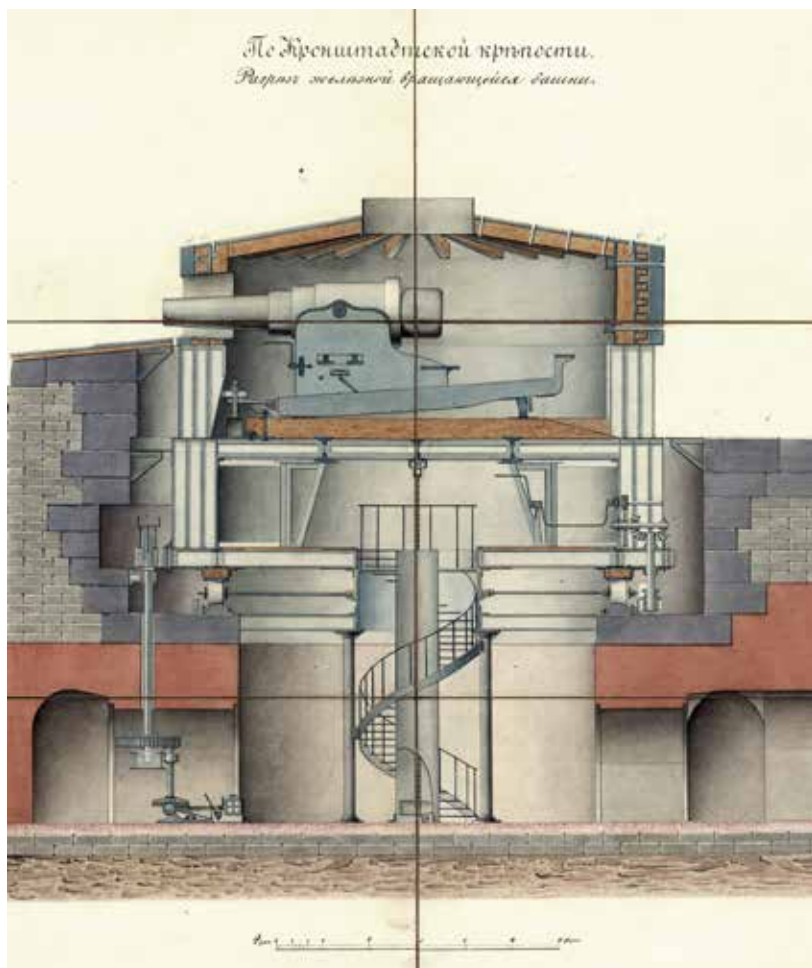
Ил. 52. Разрез по башенной установке южной морской батареи № 3. РГАВМФ. Ф. 1341. Оп. 2. Д. 308
