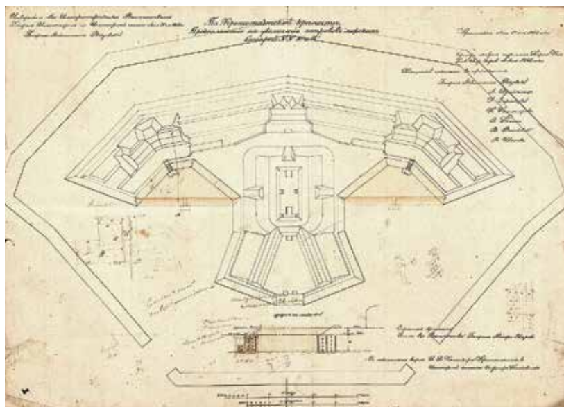
Ил. 37. Проект расширения площади островов морских батарей №№ 10 и 11. 1 июня 1866 г. РГАВМФ. Ф. 1341. Оп. 4. Д. 4871
