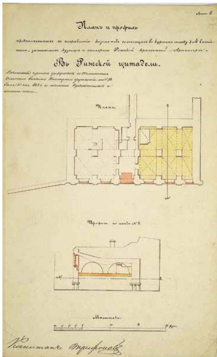
Ил. 5 Ф. 27 К-ка Крепости и Укрепления № 1 Д. 486. План и профиль предполагаемых к исправлению казематов, состоящих в куртине между 3 и 4 бастионами, занимаемых кузницею и столярною Рижской крепостной артиллерии в Рижской цитадели
