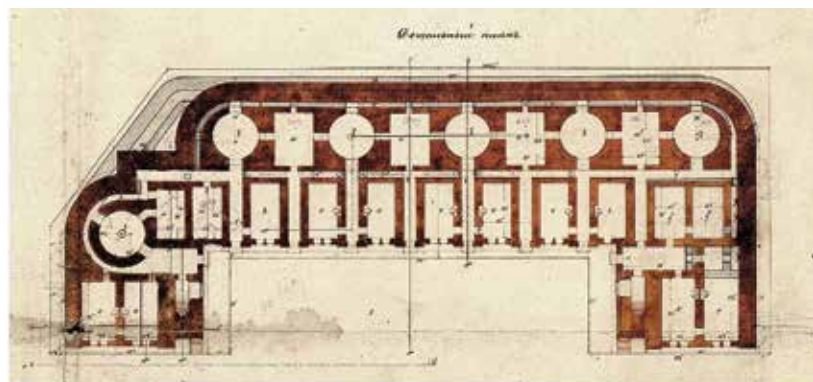
Ил. 50б. План помещений массива башенной батареи к проекту, составленному 12 апреля 1869 г. РГАВМФ. Ф. 1341. Оп. 4. Д. 6074
