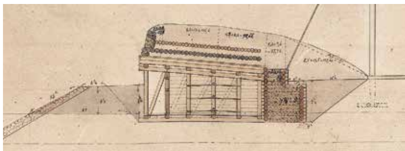
Ил. 25б. Разрез по деревокаменному блиндажу, построенному на постоянной Константиновской батарее в первую половину 1863 года. РГАВМФ. Ф. 1341. Оп. 4. Д. 4948
