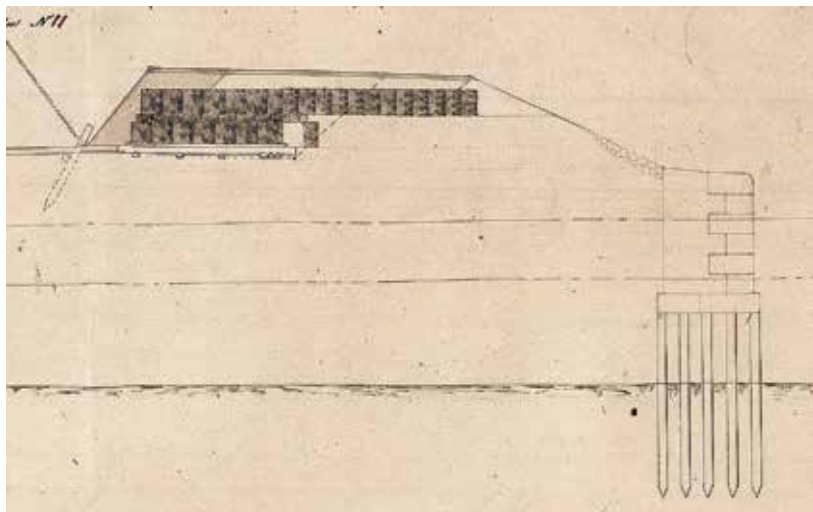
Ил. 25а. Разрез по земляному брустверу, построенному на постоянной Константиновской батарее в первую половину 1863 года. Земляные крутости бруствера укреплены фашинами. РГАВМФ. Ф. 1341. Оп. 4. Д. 4948
