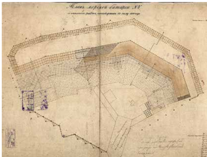
Ил. 14. План временной морской батареи № 4 ниже ординара. 1856 г. В правой части плана видны ряжевые конструкции Двойной южной батареи, а также горжевого капонира и куртин форта «Константин». РГАВМФ. Ф. 1341. Оп. 4. Д. 3864
