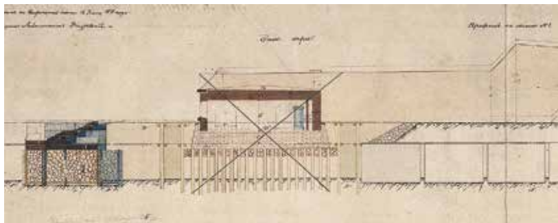
Ил. 41. Разрез по казарме в тыльной части южной морской батареи № 2 «Дзичканец». К проекту строительства казармы и порохового погреба, составленного 10 мая 1871 г. В правой части разреза схематически показаны ряжевые ящики основания временной батареи. РГАВМФ. Ф. 1341. Оп. 4. Д. 5464
