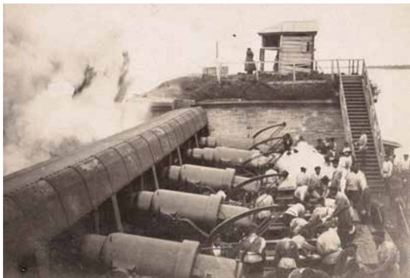
Ил. 45. Стрельба 11-дм. пушек, установленных за Колпинским броневым бруствером (запечатлен момент выстрела второго справа орудия). Фото предположительно конца XIX в. Из собрания автора
