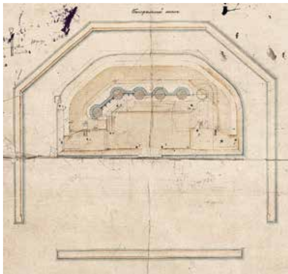
Ил. 39а. Проект морской батареи на 15 орудий в пяти броне-вых башнях и за двумя участками броне-вых брустверов. 27 февраля 1867 г. Генеральный план. РГАВМФ. Ф. 1341. Оп. 4. Д. 4852
