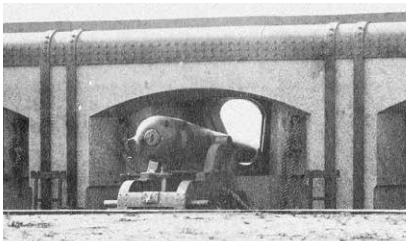
Ил. 26. 8-дм. пушка обр. 1867 г. за броневым бруствером Шведе на батарее «Константин». Фото 1869 г. Из фондов ВИМАИВиВС
