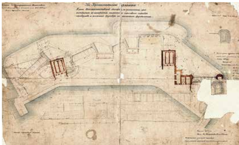
Ил. 42. Проект строительства на постоянной Константиновской батарее двух пороховых погребов, двух казематированных траверсов и пятого броневое бруствера. 30 ноября 1864 г. РГАВМФ. Ф. 1341. Оп. 4. Д. 4668
