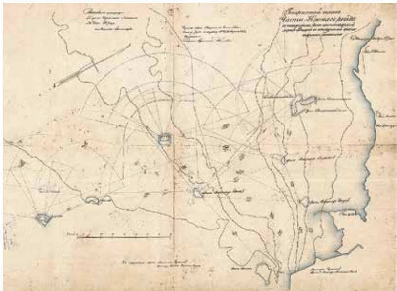
Ил. 40. «Генеральный план части Южного рейда с показанием вновь проектируемой морской батареи с железными вращающимися башнями». 13 мая 1867 г. РГАВМФ. Ф. 1341. Оп. 4. Д. 4891
