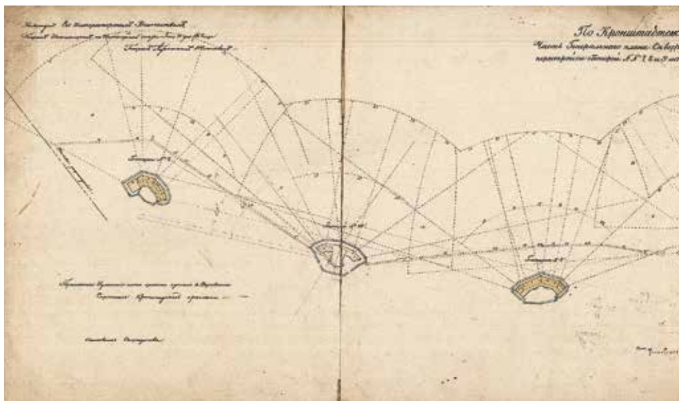
Ил. 35. Линия морских батарей №№ 7, 10, 8, 11 и 9 на Северном фарватере с нанесенной трассировкой подводного каменного заграждения. РГАВМФ. Ф. 1341. Оп. 4. Д. 4617
