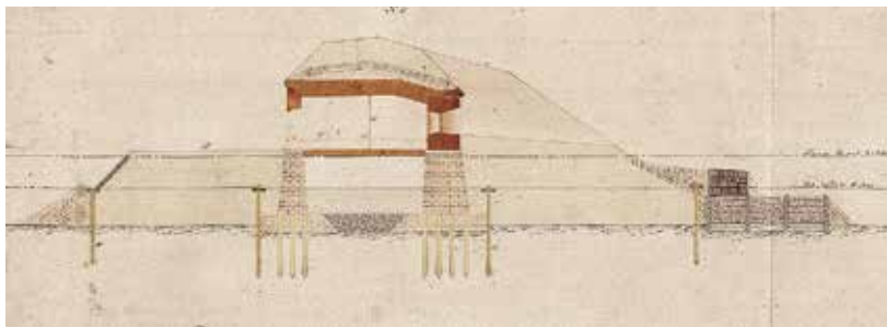
Ил. 22а. Разрез по острову и одноэтажному казематированному traversу морской батареи № 6. К проекту 1861 года. В таком виде проект реализован не был. РГАВМФ. Ф. 1341. Оп. 4. Д. 4312
