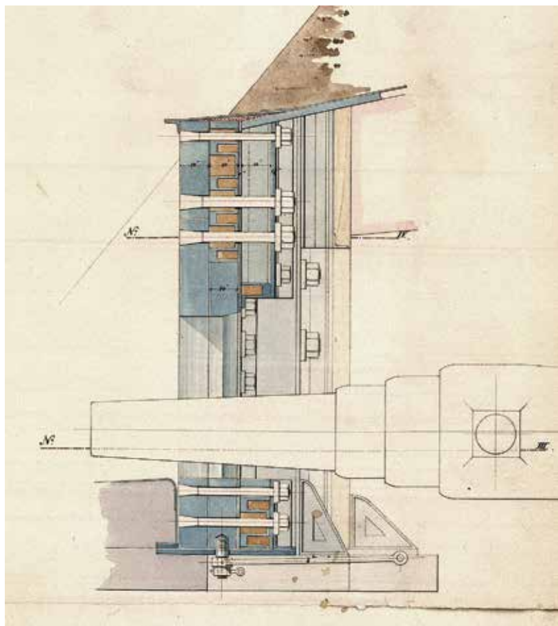
Ил. 49. Разрез по броневому амбразурному щиту казематированного траверса. 16 ноября 1869 г. РГАВМФ. Ф. 1341. Оп. 4. Д. 5126
