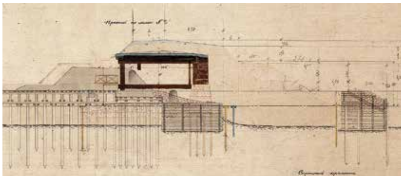
Ил. 36. Разрез по двухэтажному казематированному траверсу и эскарпу морской батареи № 1. К проекту перестройки временной батареи, составленному 20 июня 1865 г. РГАВМФ. Ф. 1341. Оп. 4. Д. 4595
