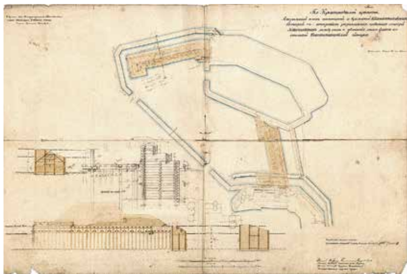
Ил. 29. «Генеральный план постоянной и временной Константиновских батарей с показанием расположения: соединения батарей Константин между собою и удлинения левого фланга постоянной Константиновской батареи». 23 января 1864 г. РГАВМФ. Ф. 1341. Оп. 4. Д. 4659
