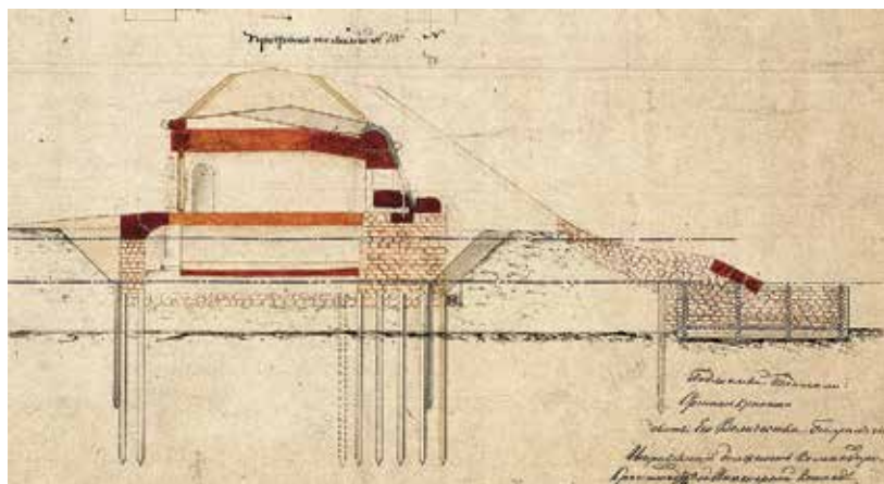
Ил. 32. Разрез по двухэтажному казематированному траверсу и эскарпу в виде наклонной гранитной вымостки к проекту перестройки морской батареи № 6. 27 марта 1864 года. На чертеже хорошо видна напольная стенка орудийного каземата, усиленная броней наподобие бруствера Шведе. (Сравните с ил. 22а.) РГАВМФ. Ф. 1341. Оп. 4. Д. 4599
