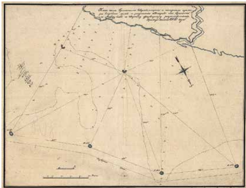
Ил. 6. План части Северного фарватера с нанесенными северными батареями (свайными и двойными). Север внизу. РГАВМФ. Ф. 1341. Оп. 4. Д. 1464
