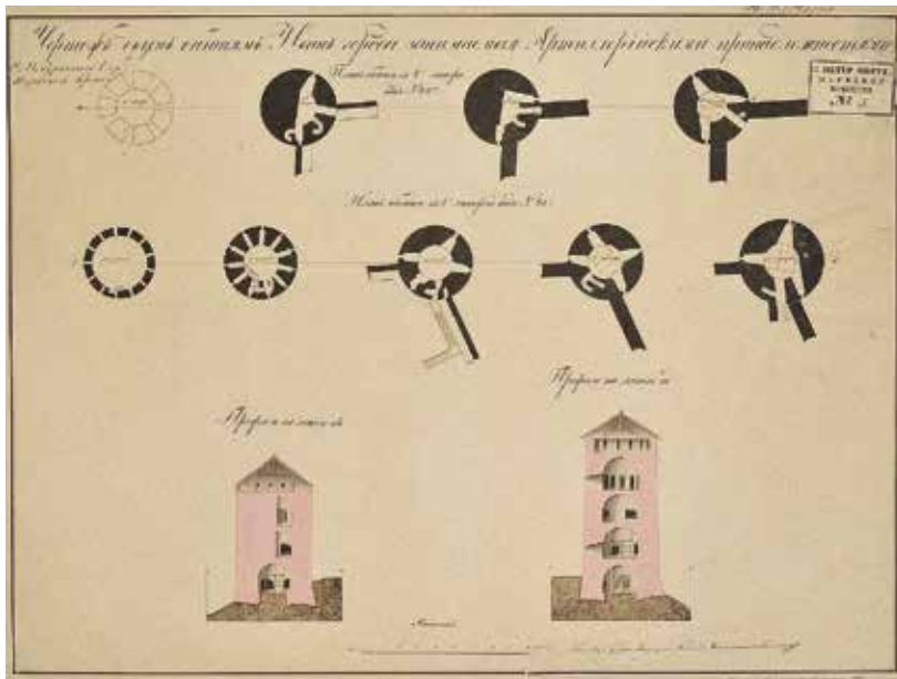
Ил. 3 Ф. 27 К-ка Крепости и Укрепления № 1 Д. 332. Чертеж двум башням Ивангорода, занимаемая Артиллерийскими принадлежностями
