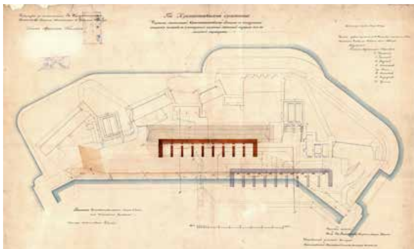
Ил. 43. Проект строительства на постоянной Константиновской батарее одноэтажной казематированной казармы. Одобрен Техническим комитетом ГИУ 10 февраля 1866 г. На чертеже показаны два варианта положения казармы: изначально предложенный (в центре) и принятый (в правой части). РГАВМФ. Ф. 1341. Оп. 4. Д. 4926
