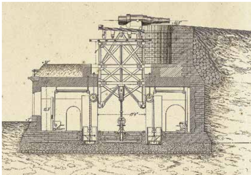
Ил. 48. Разрез по казематированной постройке для 11-дм. пушек на подъемных станках ген. Паукера. Орудие поднято в боевое положение. Атлас чертежей для руководства при составлении проектов фортификационных сооружений. 1873 г. Центральный государственный исторический архив Украины. Ф. 1436. Оп. 1. Д. 13. Л. 3
