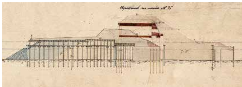
Ил. 31а. Разрез по казематированному траверсу к проекту перестройки временной морской батареи № 9. Бывший ряжевый волнолом (на разрезе справа) обращен в эскарпную стенку. Бывшая ряжевая стенка попала под основание казематированного траверса. РГАВМФ. Ф. 1341. Оп. 4. Д. 4627
