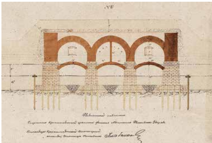
Ил. 22 в. Продольный разрез по одноэтажному казематированному traversу морской батареи № 6. К проекту 1861 года. РГАВМФ. Ф. 1341. Оп. 4. Д. 4312
