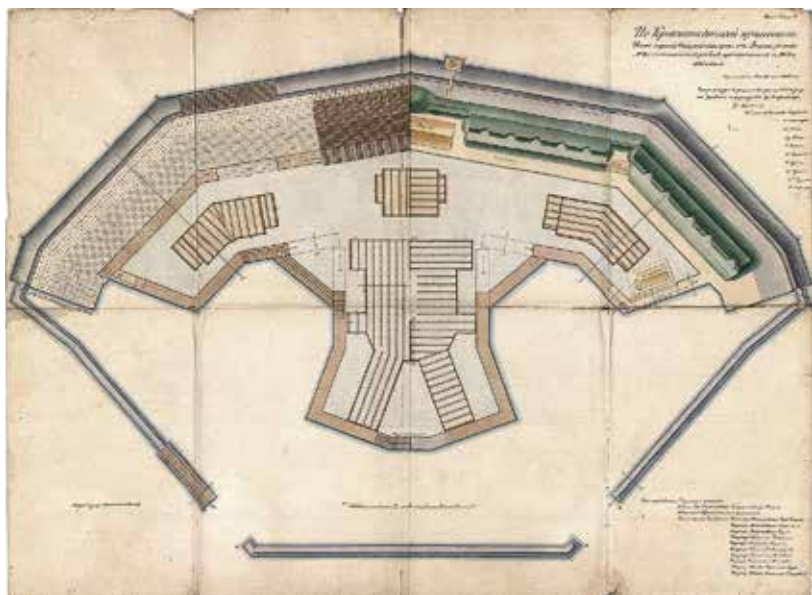
Ил. 33. План морской батареи № 10, показывающий работы, произведенные в 1864 и 1865 годах. В левой части показано сплошное свайное поле во рву между эскарпом и волноломом, в правой части этого же рва — временная земляная позиция для артиллерии. РГАВМФ. Ф. 1341. Оп. 4. Д. 5139
