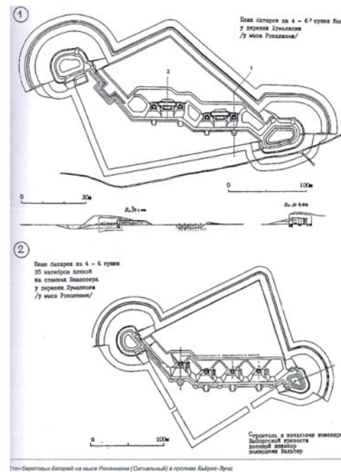
Ил. 2. Российский чертеж береговых батарей у д. Хумалиоки. Изображение из статьи С. Прямыцкого «Приморская крепость Выборг (1710–1918)»
