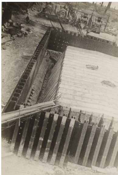
Ил. 5. Засыпка грунта между внутренним и наружным каркасами. Вдали виден бетонный завод и 7,5-тонный кран
