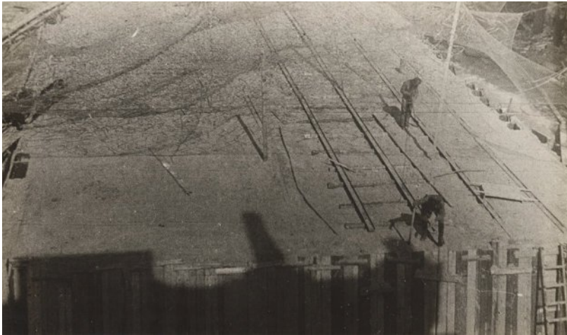
Ил. 8. Укладка монтажных путей по перекрытию сооружения для перемещения бронеплит. Над местом проведения работ растянута маскировочная сеть. На переднем плане хорошо видны доски, при помощи которых заделаны промежутки между шпангоутами срубов. Это сделано для того, чтобы тюки с хлопком, которыми обкладывалось сооружение, не проваливались внутрь
