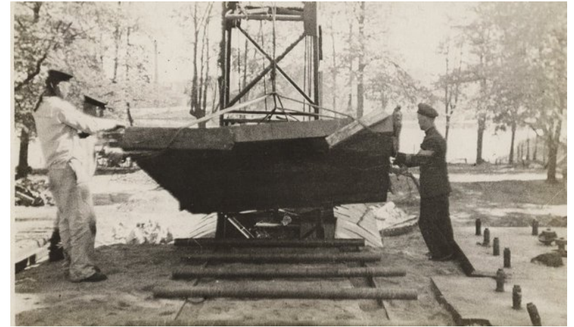
Ил. 9. Момент подъёма краном бронеплиты на металлические катки. Как видно на фотографии, в качестве рельсового пути использовались двутавровые балки, уложенные на шпалы. После монтажа всей поверхности покрытия сооружения они так и остались на своих местах. Плиту придерживают краснофлотцы, одетые в рабочие робы
