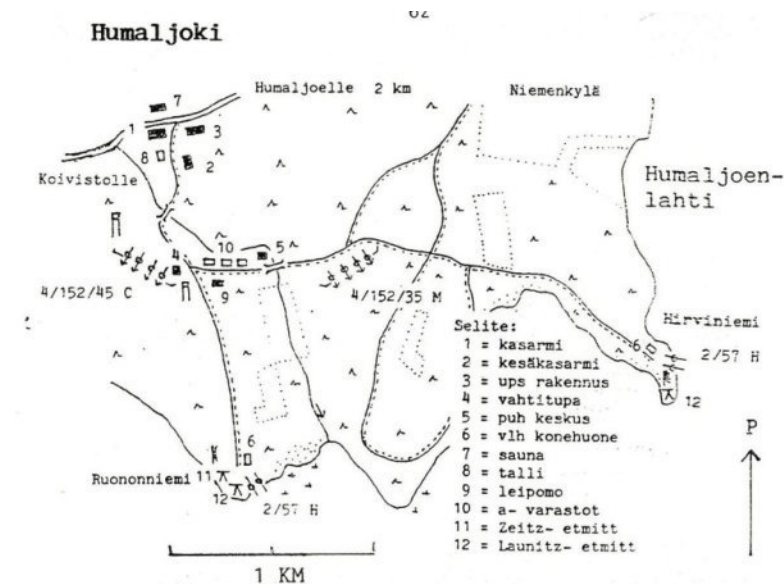
Ил. 3. Финская схема расположения сооружений форта Хумалиоки. Изображение из книги Rannikkotyökirjasto 2. 1918–1940.
