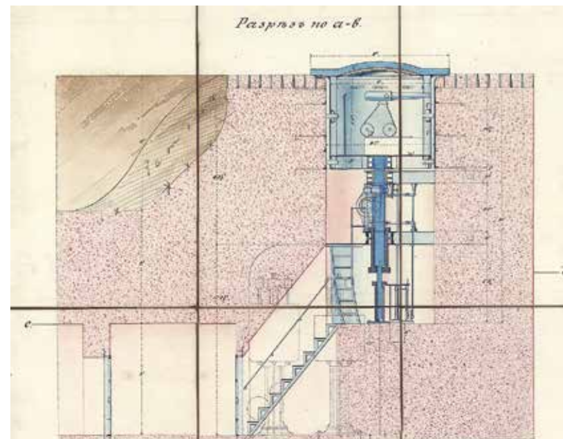
Ил. 5. Проектный чертёж скрывающейся броневой башни с гидравлическим устройством подъёма. 1891 г. РГАВМФ. Ф. 1341. Оп. 2. Д. 268
