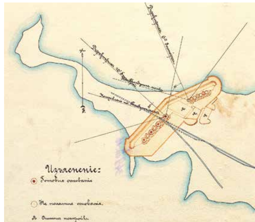
Ил. 12. Чертёж батареи «Риф» на четыре 10-дюймовые пушки и четыре 6-дюймовые пушки Канэ согласно проекту, утверждённому 3 сентября 1909 г. РГВИА. Ф. 349. Оп. 16. Д. 5168
