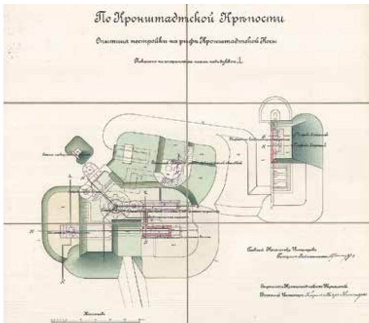
Ил. 6. Общий план опытных построек на рифе Кронштадтской косы к отчёту о работах в 1897 г. Справа — восточная группа сооружений с прусскими казематами. РГАВМФ. Ф. 1341. Оп. 3. Д. 580. Л. 2
