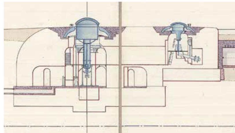
Ил. 7. Фрагмент отчётного чертежа по работам 1897 г. РГА ВМФ. Ф. 1341. Оп. 3. Д. 580. Л. 1
