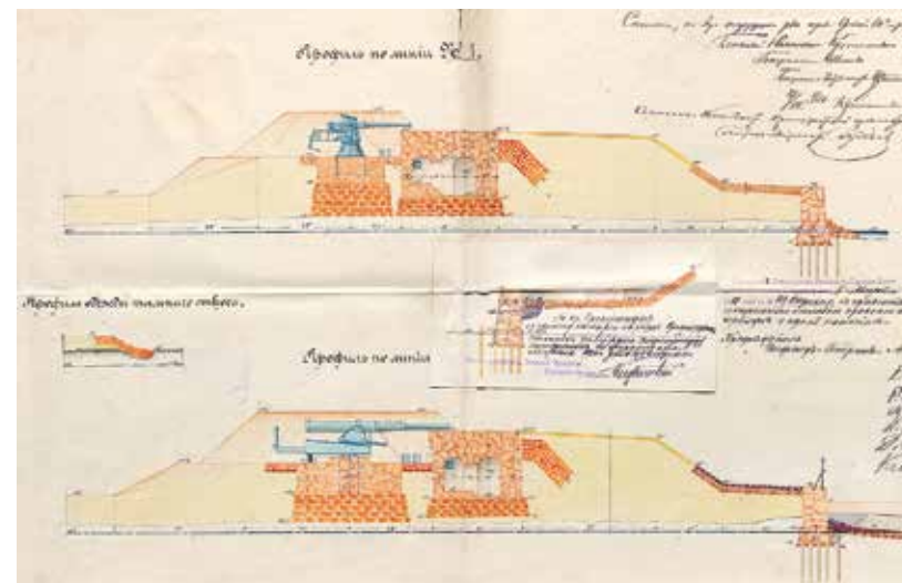
Ил. 13б. Профили по орудийным дворикам с 6-дюймовыми (вверху) и 10-дюймовыми орудиями. РГВИА. Ф. 349. Оп. 16. Д. 5267
