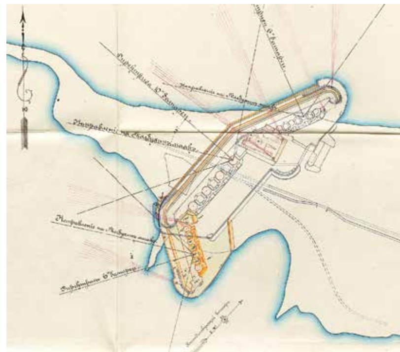
Ил. 14. Проект левофланговой 6-дюймовой батареи на рифе Кронштадтской косы, утверждённый 11 февраля 1910 г. РГВИА. Ф. 349. Оп. 16. Д. 5255
