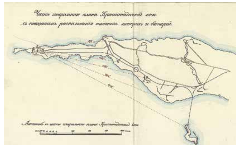
Ил. 3. Схема острова Котлин, показывающая положение опытных построек на рифе Кронштадтской косы и батарей, с которых производился их обстрел. РГАВМФ. Ф. 1341. Оп. 3. Д. 597
