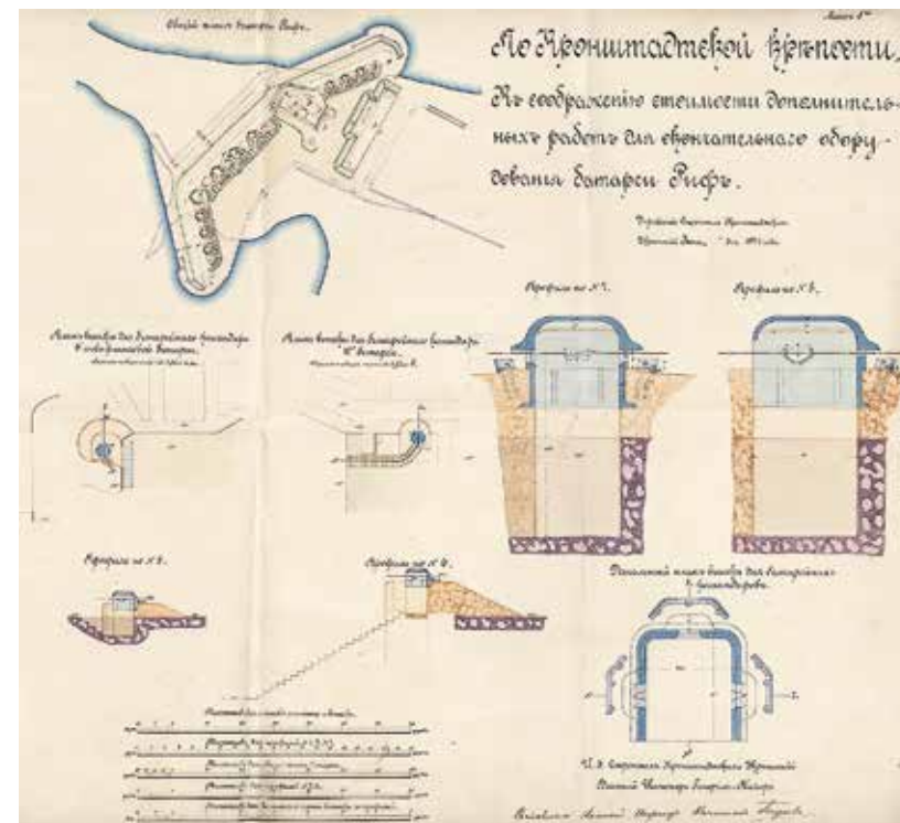
Ил. 16. Фрагмент проекта дополнительных работ на батарее «Риф», составленный в июне 1911 г. РГАВМФ. Ф. 1341. Оп. 3. Д. 375
