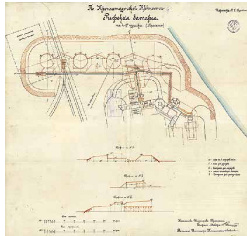
Ил. 11. Проект временной батареи на четыре 11-дюймовые пушки на рифе Кронштадтской косы. Начало 1905 г. РГАВМФ. Ф. 1341. Оп. 2. Д. 371
