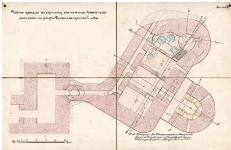
Ил. 4. Проектный план каземата «Ж» с гидравлической башней и капониром «З». 1891 г. РГАВМФ. Ф. 1341. Оп. 2. Д. 272
