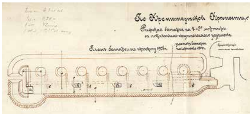
Ил. 10. План Рифской mortarной батареи с учётом модернизации в 1905 г. РГАВМФ. Ф. 1341. Оп. 2. Д. 367
