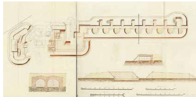
Ил. 9. Проект передового укрепления на рифе Кронштадтской косы с временной батареей на восемь 9-дюймовых мортир. 1904 г. РГАВМФ. Ф. 1342. Оп. 2. Д. 1912. Л. 3, 8
