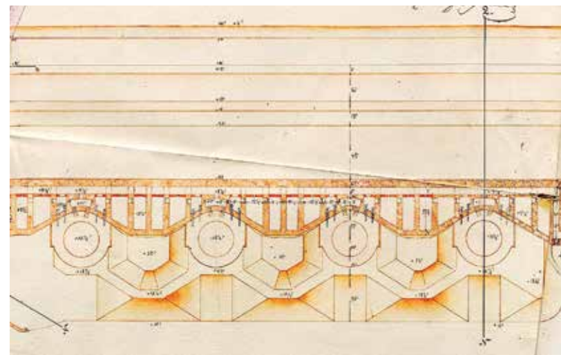
Ил. 13а. Детальный план 10-дюймовой батареи на рифе Кронштадтской косы. РГВИА. Ф. 349. Оп. 16. Д. 5266
